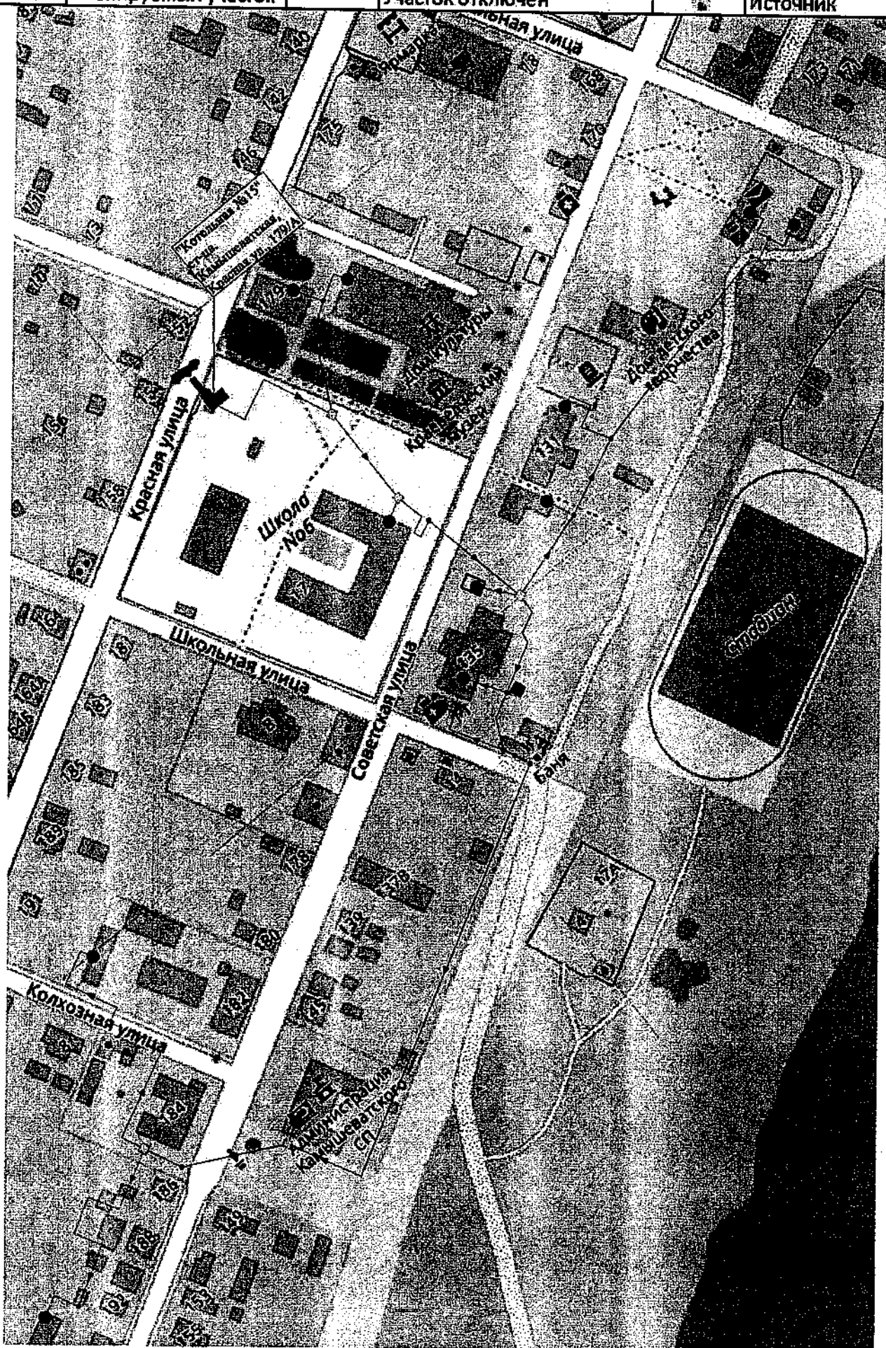
Схема тепловых сетей – котельная № 15 в ст-це Камышевской по ул. Красной, 179/А
